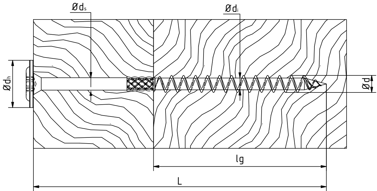
Vue latérale
