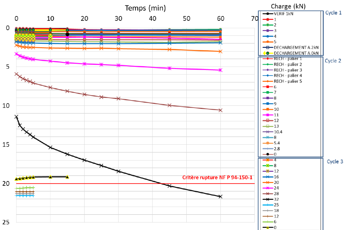
ESSAI FINAL - Vis 60-750 - Enfoncement en fonction du temps par palier de chargement
